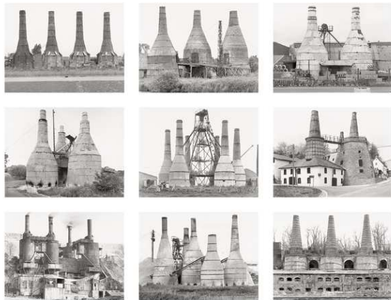
8) Kalköfen (Typologie), 1963-1994
